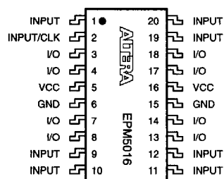
SOIC
