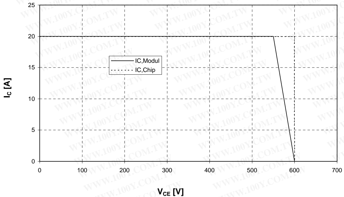
Sicherer Arbeitsbereich Wechsler. (RBSOA) I_c = f(V_{CE}) Reverse bias safe operating area Inverter (RBSOA) T_{vj} = 125^\circ\text{C} , V_{GE} = \pm 15\text{V} , R_G = 82\ \Omega
