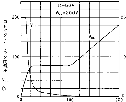
ゲート電荷 Q_g (nC) ゲート電荷(標準値)
