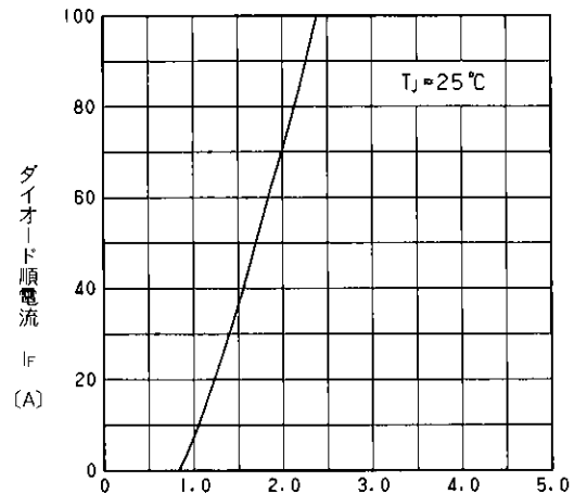
ダイオード順電圧 V_f (V)
