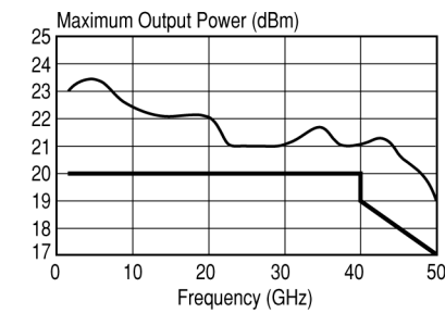
83050A Amplifier
