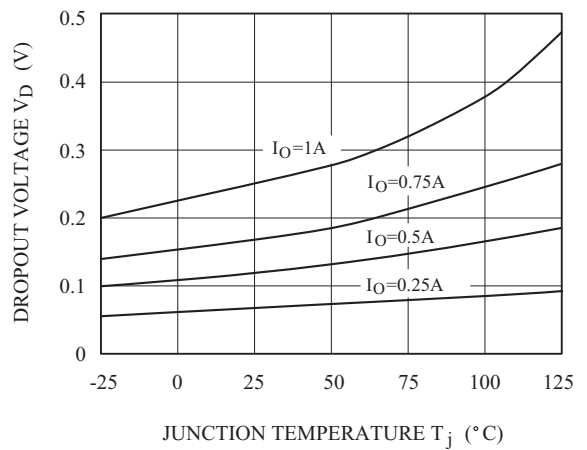
Fig.9 T_j - V_D
