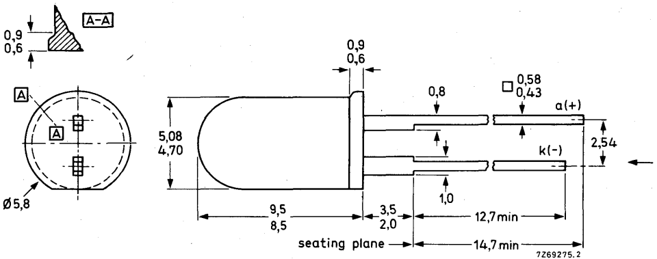
Fig. 1 SOD-63.
