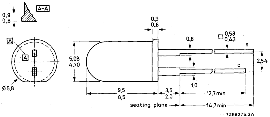
Fig. 1 SOD-63.
