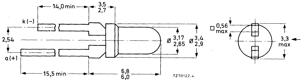
Fig. 1 SOD-53C.
